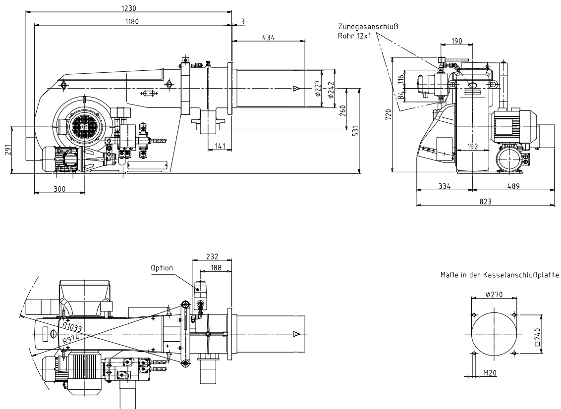
Maßbild EK 6.170 / 200 GL-EU
