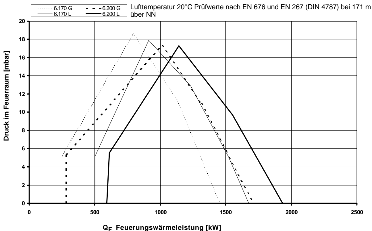
Arbeitsfeld EK 6.170 / 200 GL-EU
