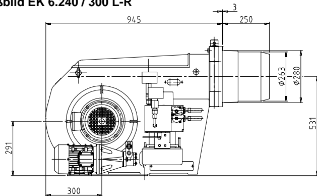
Maßbild EK 6.240 / 300 L-R
