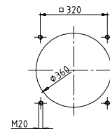
Maße in der Kesselanschlußplatte
