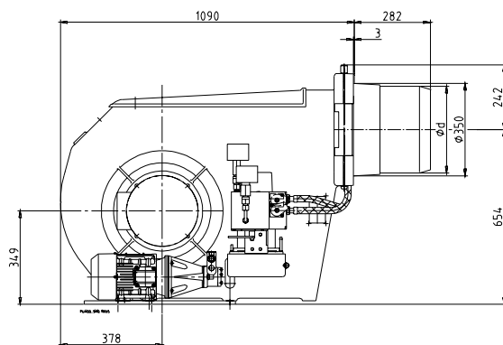
Maßbild EK 7... L-R
