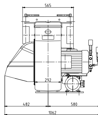
Maße in der Kesselanschlußplatte
