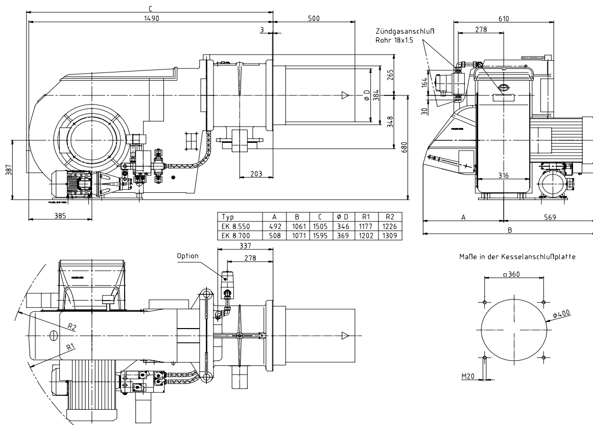
Maßbild EK 8... GL-EU
