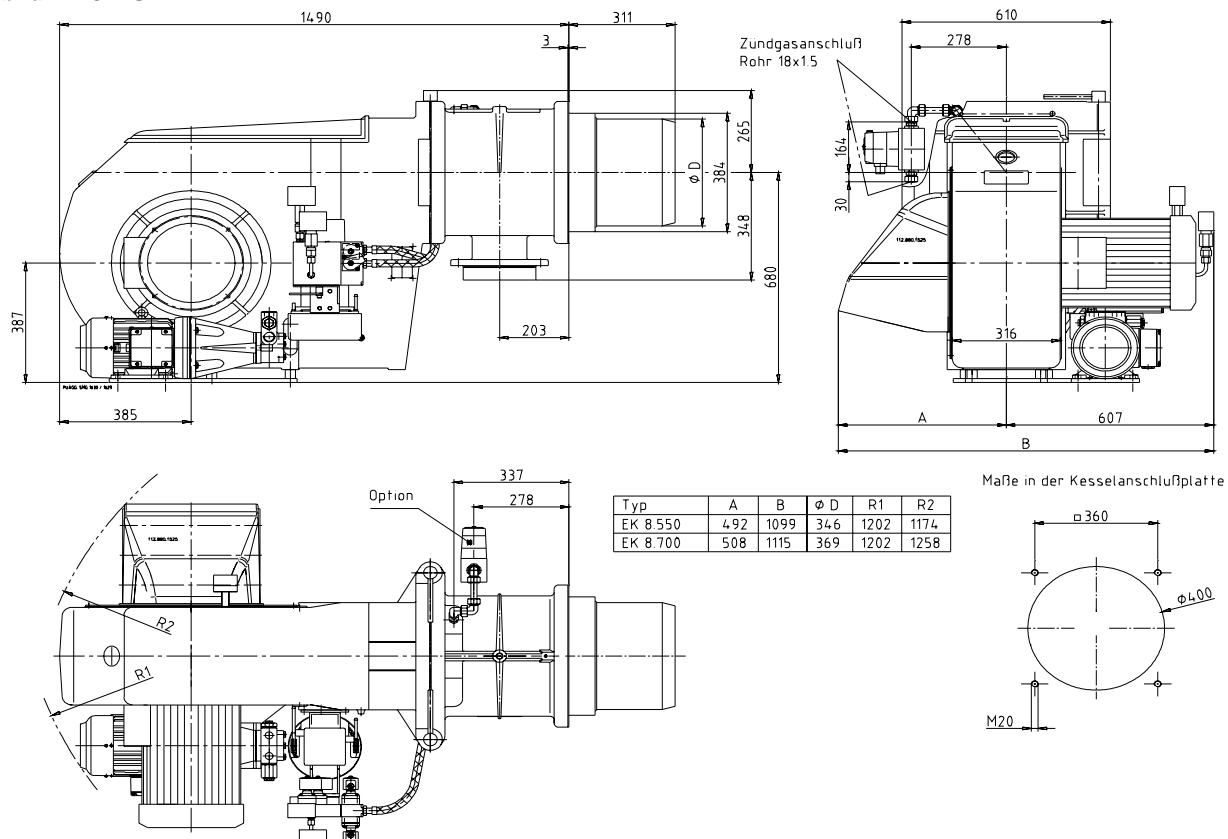
Maßbild EK 8... GL-R
