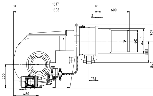
Maßbild EK 9... GL-EU
